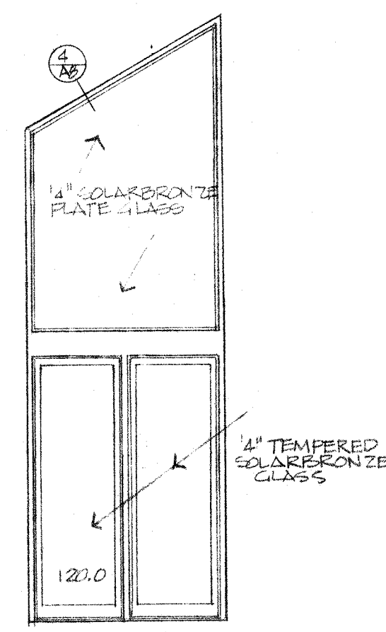
11 A10 DOOR 120.3 SCALE 1/4\"/>
